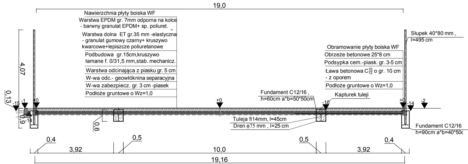
PRZEKRÓJ KONSTRUKCYJNY PŁYTY BOISKA WIELOFUNKCYJNEGO, CICHE DZ. NR 301/12
